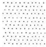
fine
